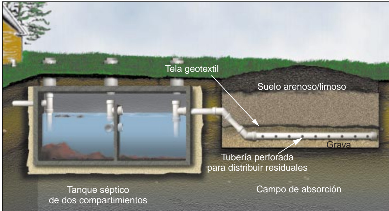
Figura 1: Una fosa séptica y un sistema de campo de absorción.
