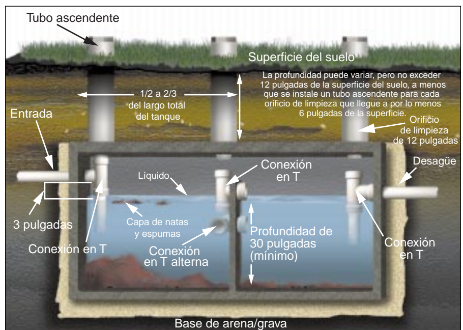
Figura 2: Una fosa séptica de dos compartimientos.
